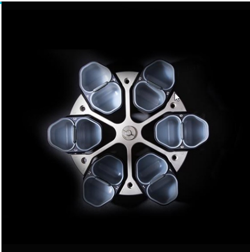
Арт. 4176. 6-местный горизонтальный ротор
